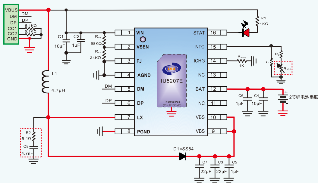
IU5207E应用电路图
