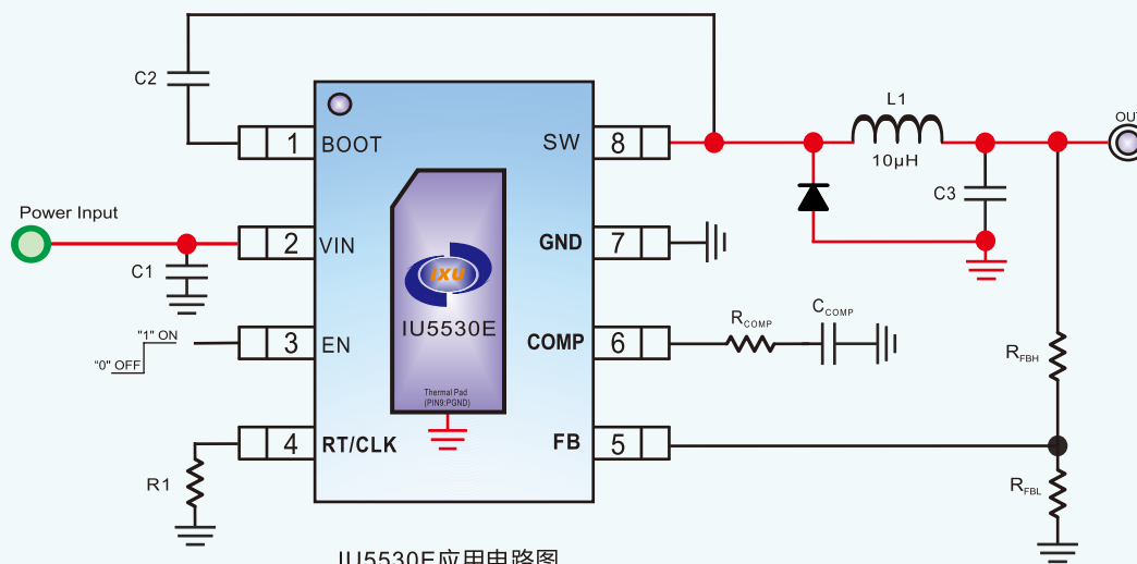
IU5530E应用电路图
