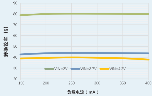
转换效率 vs. 负载电流
