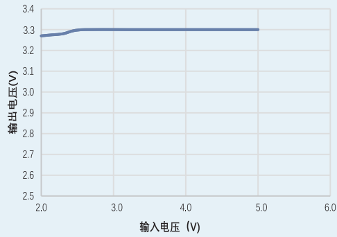
输出电压 Vs. 输入电压 (负载电流=0mA)
