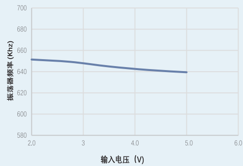
振荡器频率 Vs. 输入电压 (负载电流=100mA)
