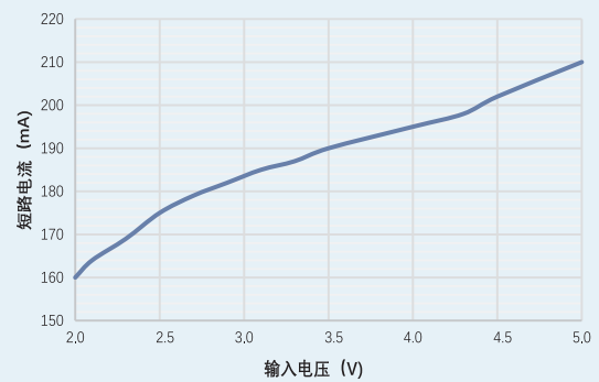
输出短路电流 Vs. 输入电压
