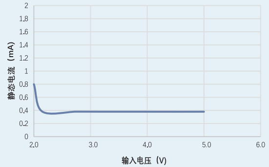
静态电流 Vs. 输入电压 (负载电流=0mA)
