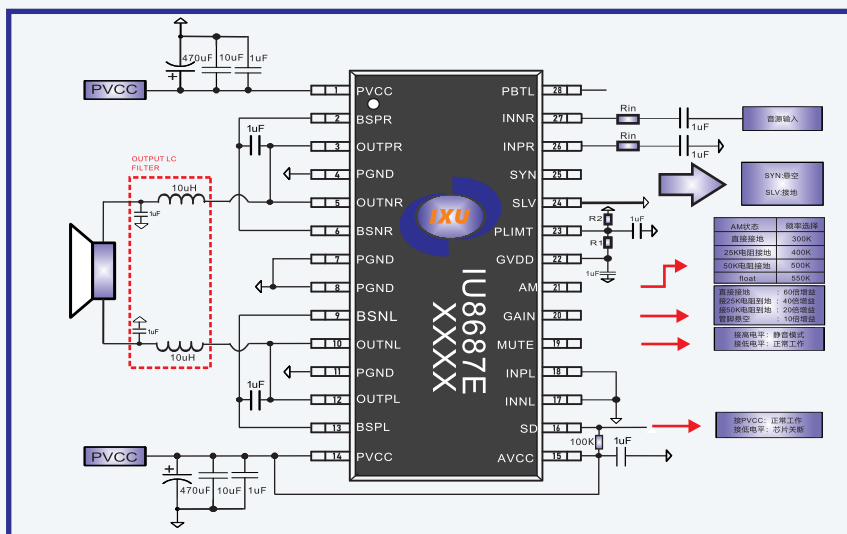
IU8687E PBT 模式应用图
