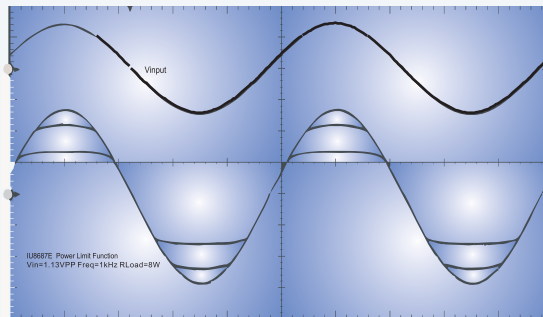
IU8687E功率限制波形
