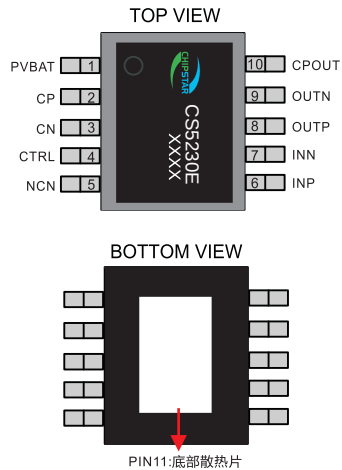
CS5230E ESOP10 PACKAGE)
