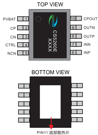
CS5260E(ESOP10 PACKAGE)
