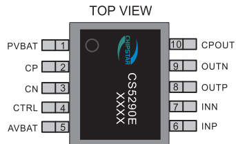
CS5290E(ESOP10 PACKAGE)
