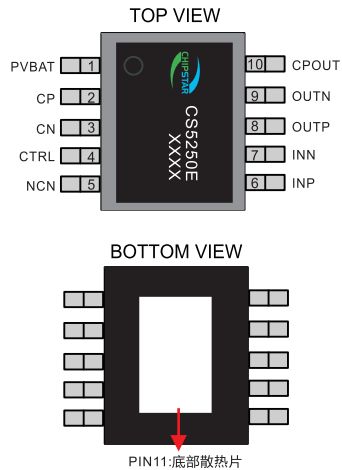
CS5250E(ESOP10 PACKAGE)
