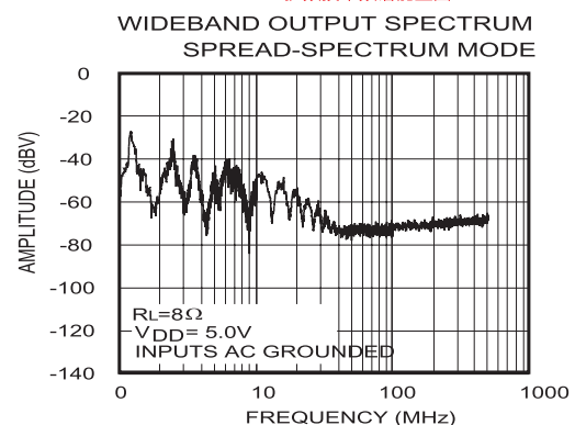
CS8631E 扩频技术频谱能量图
