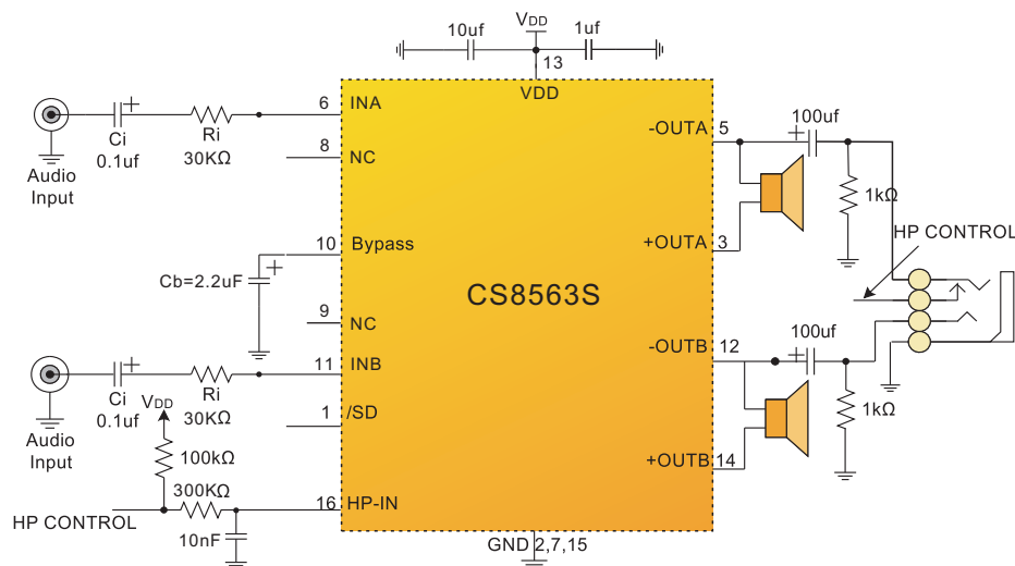
图 1 CS8563S 应用线路图
