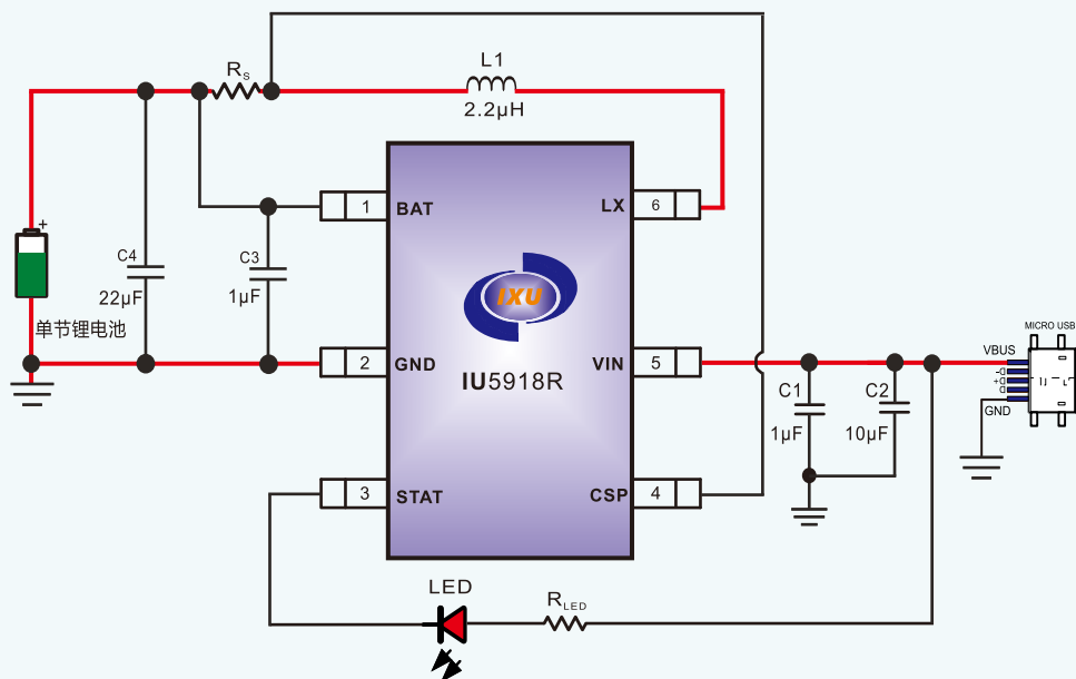
IU5918R应用电路图
