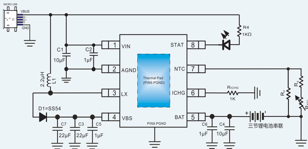
CS5095EA应用电路图
