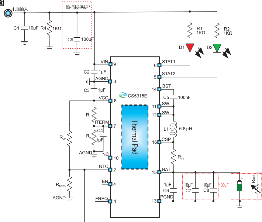
CS5315E应用电路图
