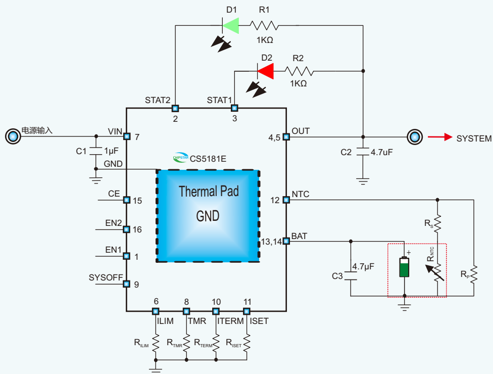
CS5181E应用电路图
