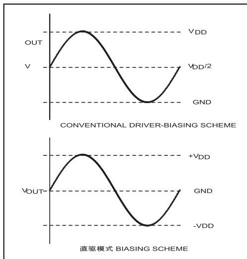
图1. 传统的驱动器输出波形与CS5012S的输出波形
