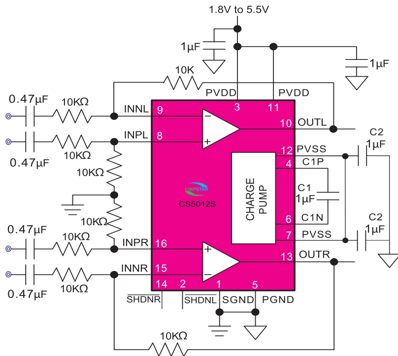
CS5012S应用电路图
