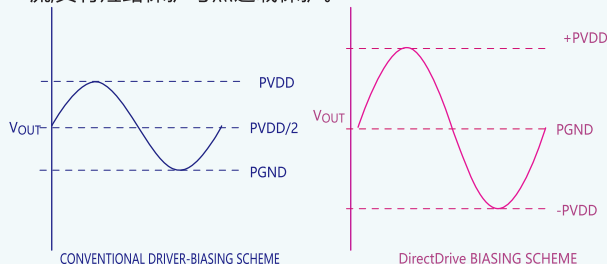
图1. 传统的驱动器输出波形与IU8202T的输出波形
