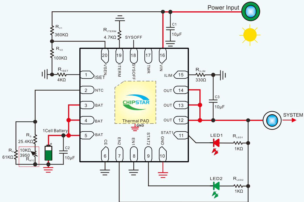
CS5160D对200mAH电池充电应用电路图
