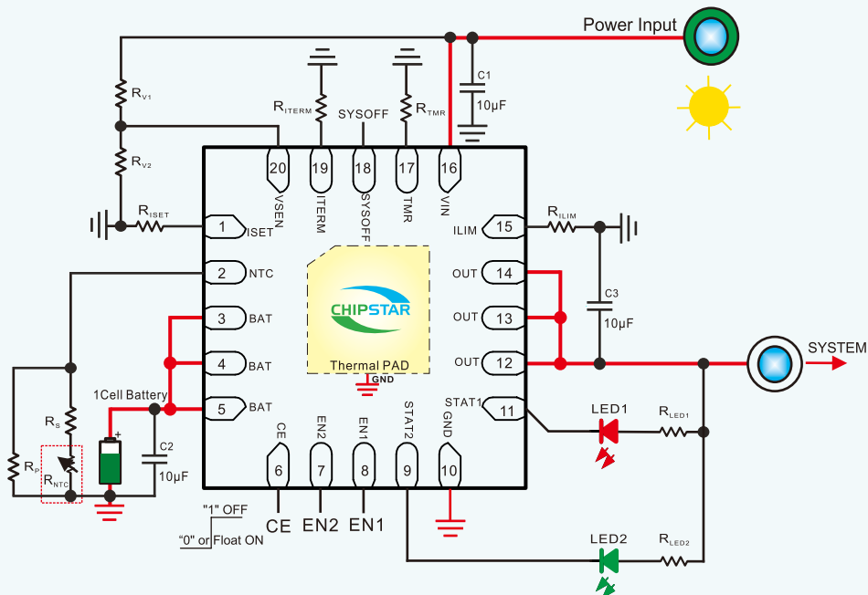
CS5160D应用电路图
