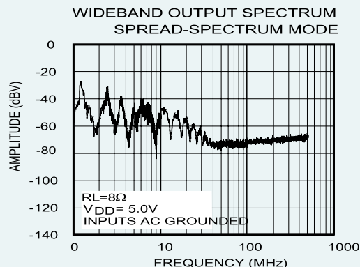
IU8632E 扩频技术频谱能量图
