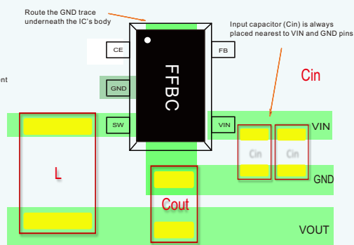
图2. PCB LAYOUT推荐
