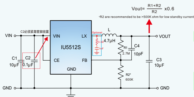
图1. 应用图
